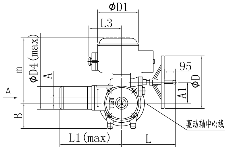
QBR3. IN~QBR5. IN系列外形尺寸
